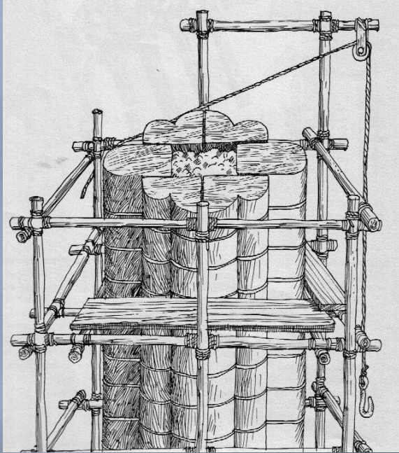
Pilastro gotico a fascio
