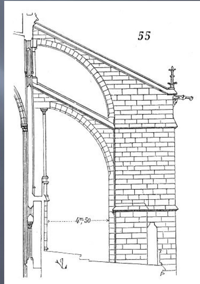
Arco rampante
