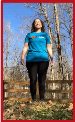
Scalene
