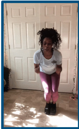
Isosceles
