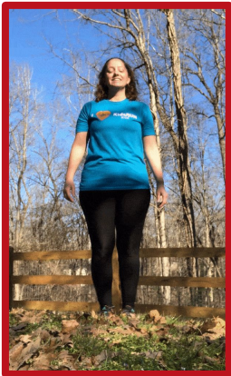
Scalene
