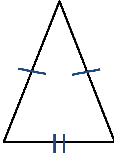
Isosceles
