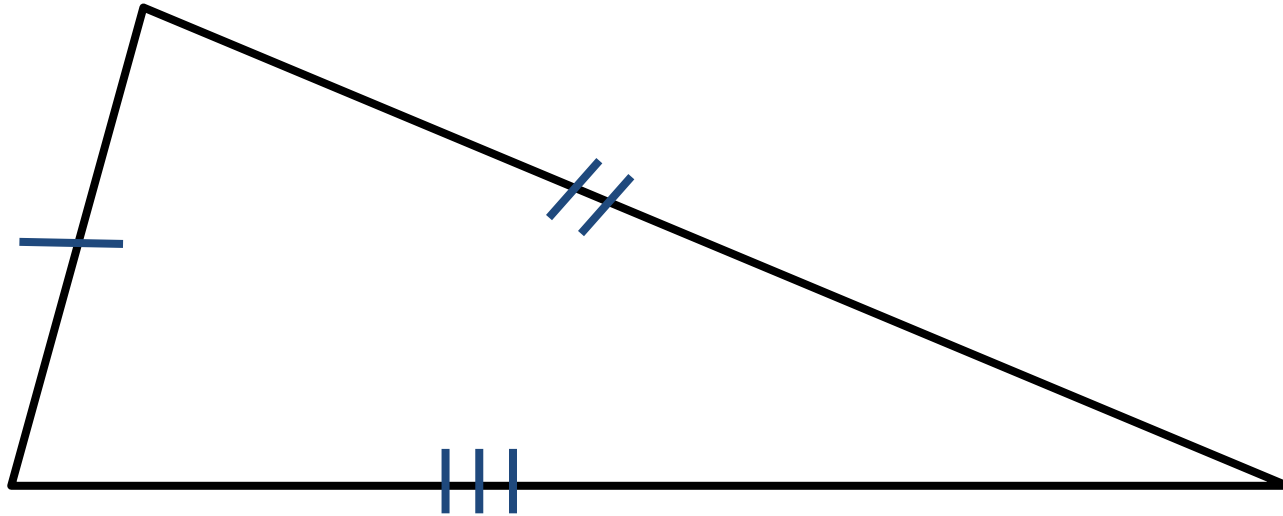
Scalene
