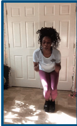
Isosceles
