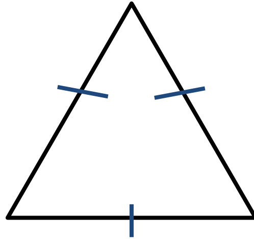
Isosceles
