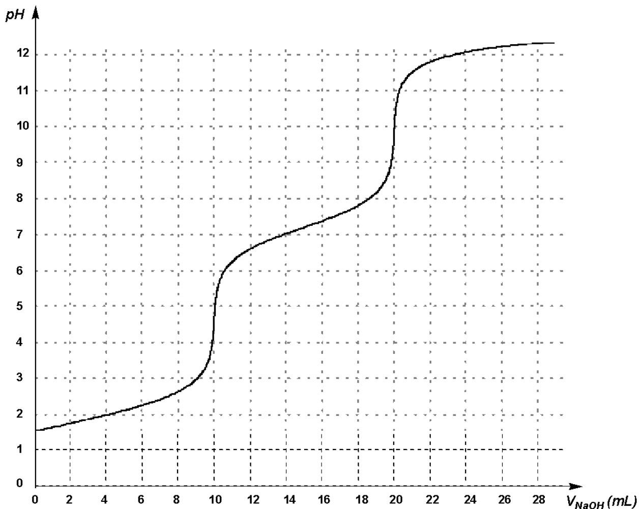
Courbe de dosage d'une solution de \text{SO}_2(\text{aq}) par une solution aqueuse de soude
