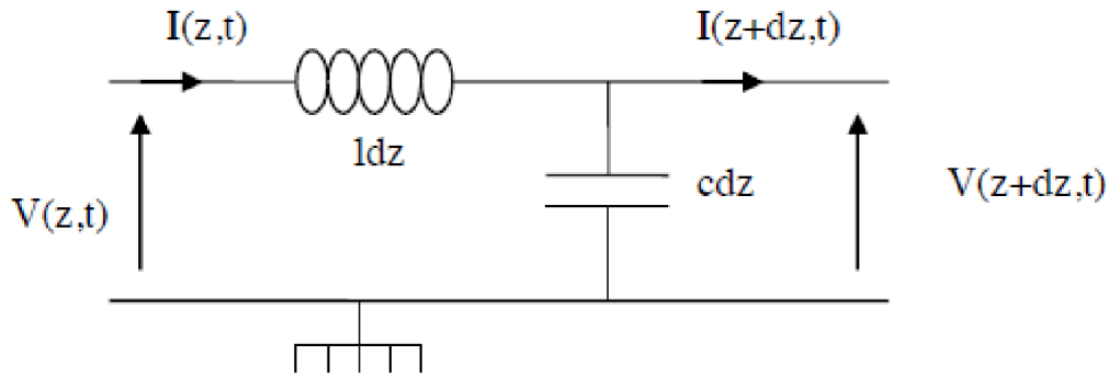
Figure 9 : modèle réparti
