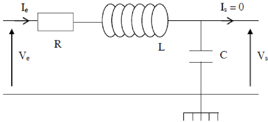
Figure 8 : modèle global de ligne électrique courte
