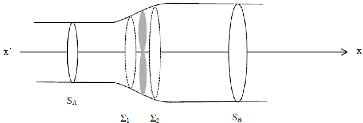
Figure 5 : pales de l'éolienne et tube de courant
