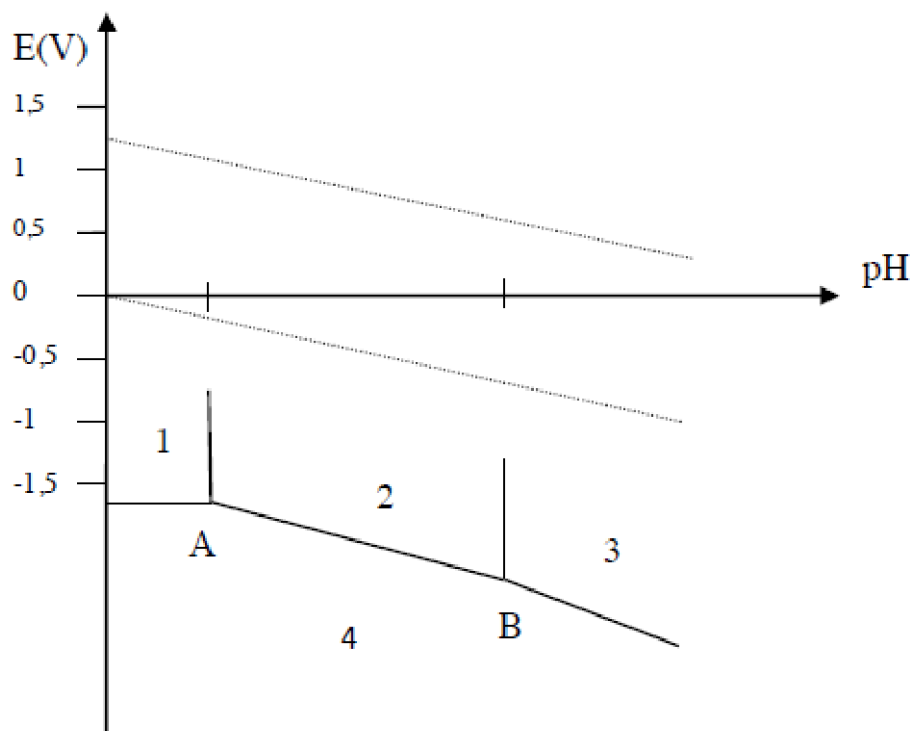
Figure 2 : diagramme E-pH de l'aluminium
