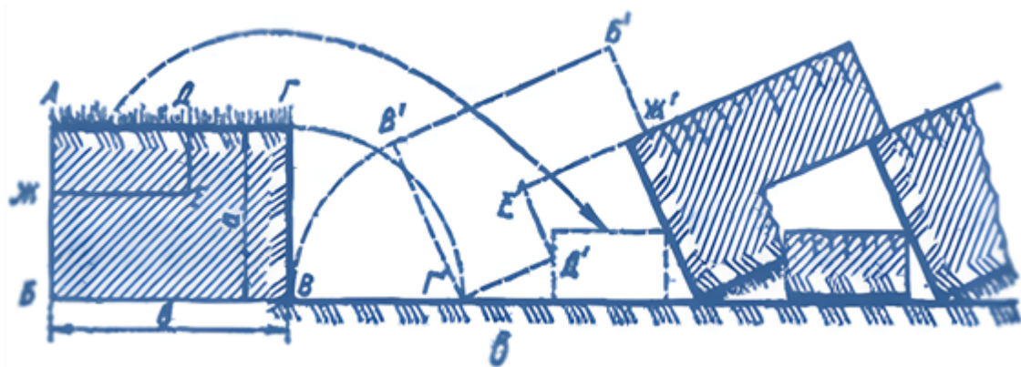
Рис. 1.2.9. Схема перевертання скиби
