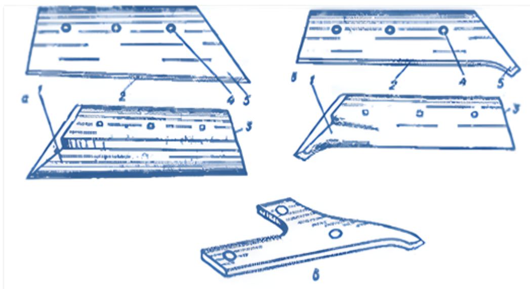
Рис. 1.2.4. Типи лемешів:
