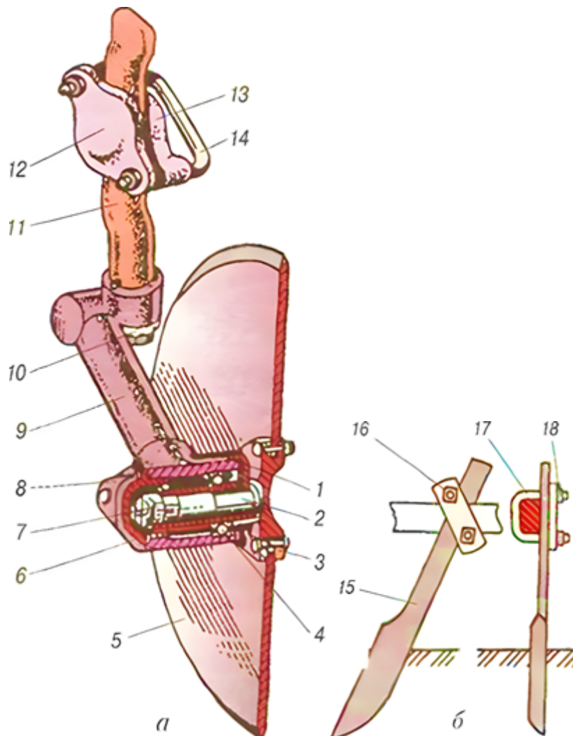
Рис. 1.2.7. Ножі:
