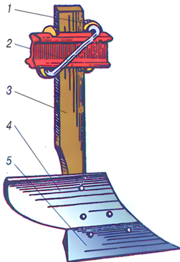
Рис. 1.2.6. Передплужник:
