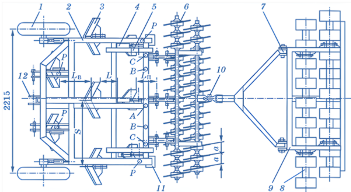
Рис. 1.2.14. Схема розпушувача для різноглибинного обробітку ґрунту РПН-2,5М:
