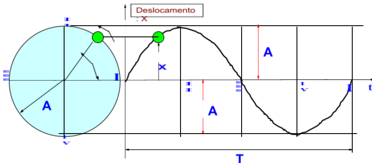
Figura 1.3 : Deslocamento de um MHS em função do tempo.
