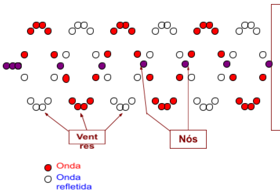
Figura 1.10: Reflexão de uma onda e formação da onda estacionária
