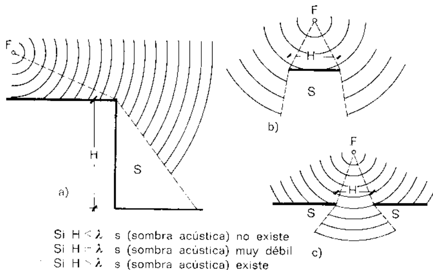
Figura 3.4 - Difração de um som agudo.
