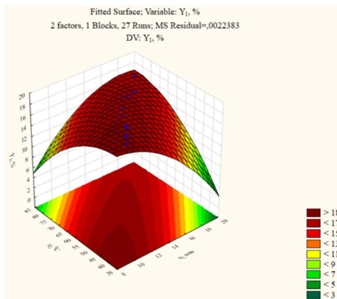
12 сурет – Y_1 үшін жауап беті: белоктың массалық үлесіне температура мен уақыттың әсері
