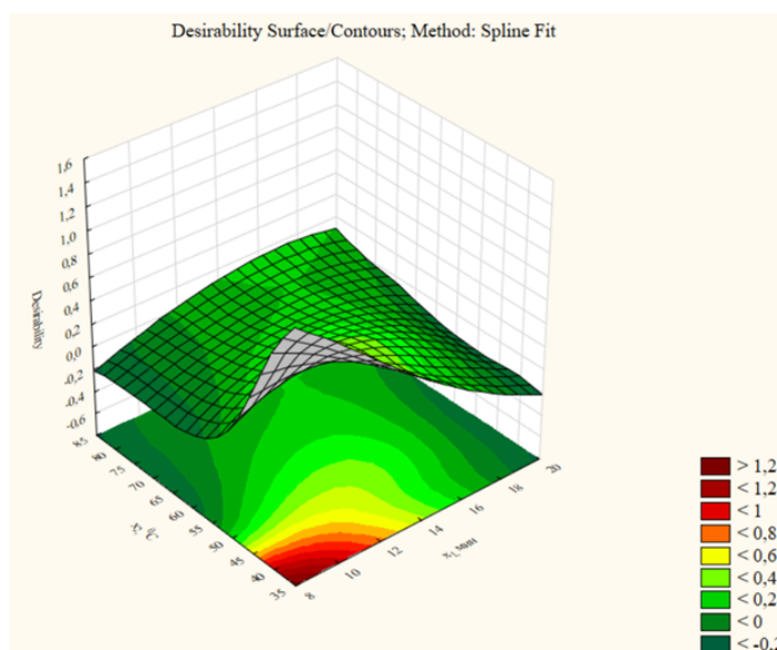
13 сурет – y_1 үшін қажеттілік графигі
