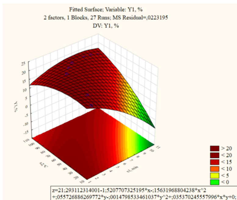
17 сурет – y_1 үшін жауап беті: белоктың массалық үлесіне температура мен уақыттың әсері
