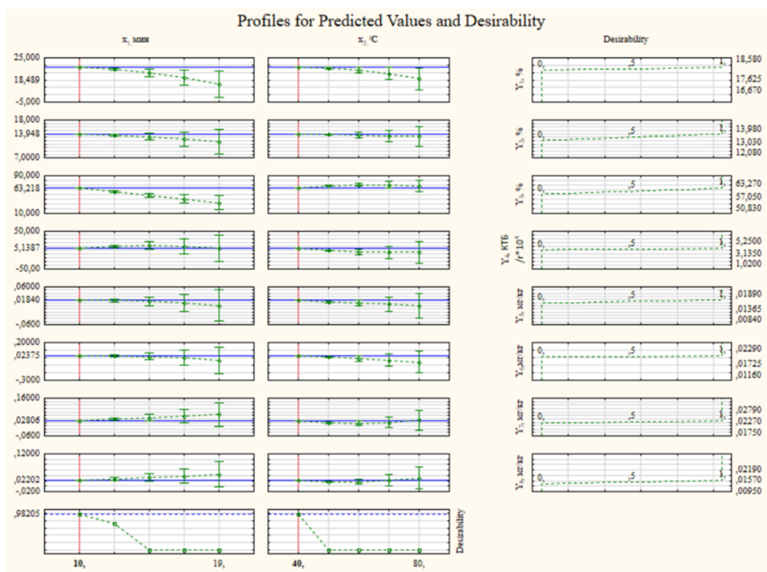
Сурет 16 – болжамды мәндер мен қалаулылық профильдерінің диаграммасы
