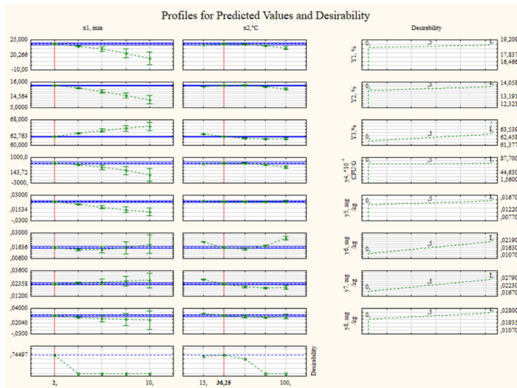
Сурет 23 – болжамды мәндер мен қалаулылық профилдерінің диаграммасы
