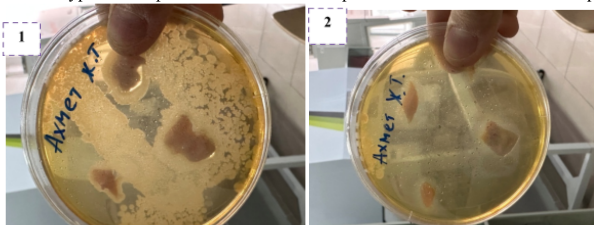
Сурет 2 – Зертхана жағдайында өсірілген Bacillus subtilis штамдары
