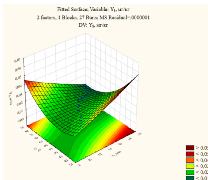
15 – сурет – y_8 үшін жауап беті: эстрадиол концентрациясына температура мен уақыттың әсері
