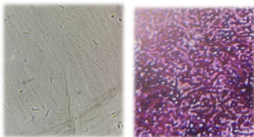
Сурет 2 – Зертхана жағдайында өсірілген Bacillus subtilis штамдары
