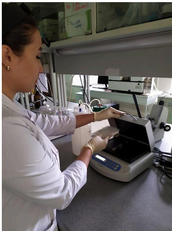
Сурет Г.1 – ИФА талдау жүргізу барысы
