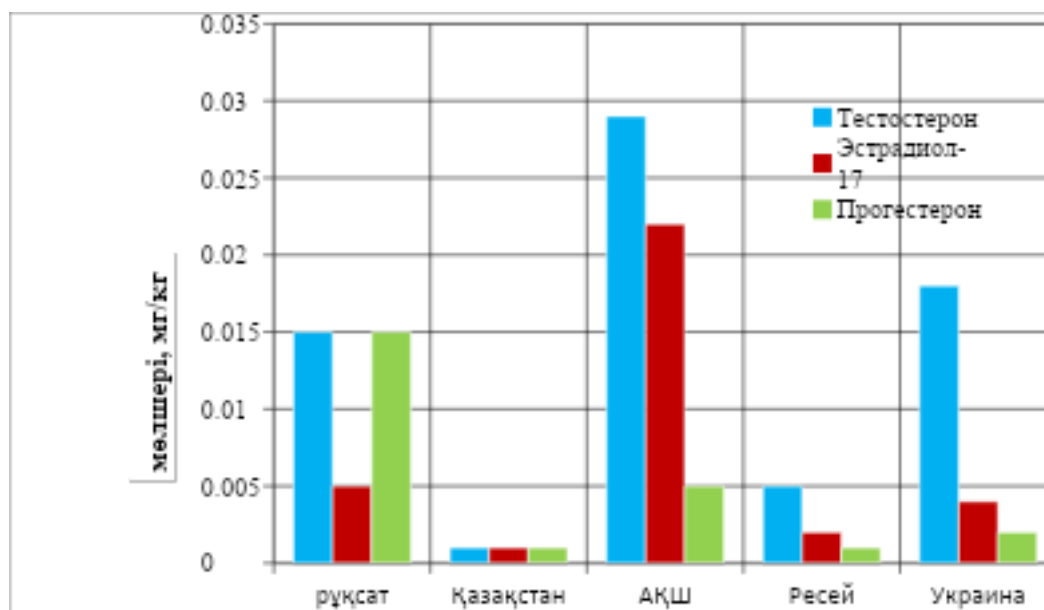
Сурет 7 – Гормоналды өсу стимуляторлары қалдығын анықтау нәтижесі
