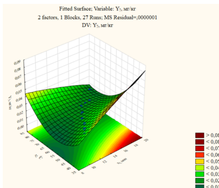
14 сурет – y_7 үшін жауап беті: тестостеронның концентрациясына температура мен уақыттың әсері
