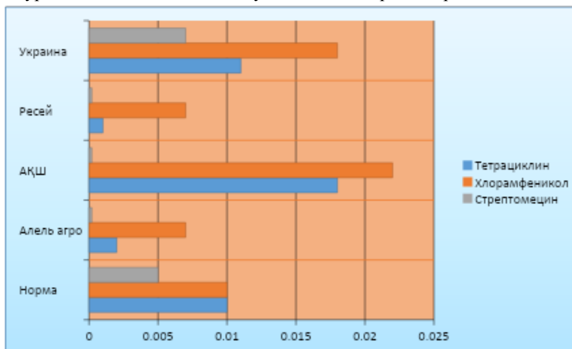
Сурет 5 – Антибиотик анықтау нәтижесінің хроматограммасы
