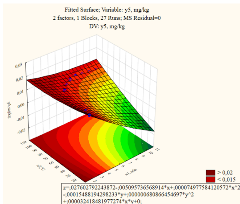
20 сурет – y_5 үшін жауап беті: тетрациклиннің концентрациясына температура мен уақыттың әсері
