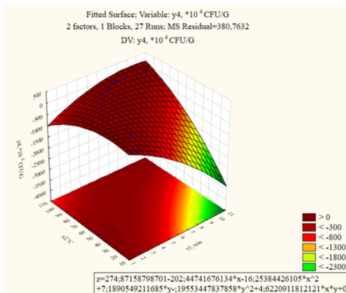
19 сурет – y_4 үшін жауап беті: мезофильді аэробы және факультативті анаэробты микроорганизмдер санына температура мен уақыттың әсері
