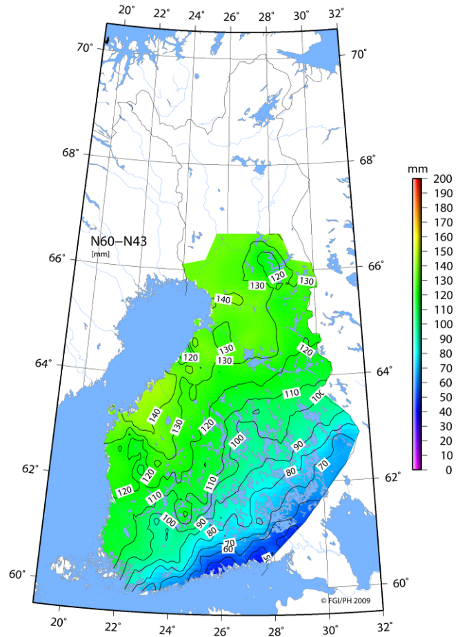
Kuva 4: N60-N43 muunnosarvot ( H_{N60} - H_{N43} ) [mm]
