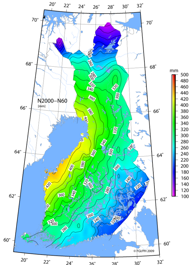
Kuva 2: N2000-N60 muunnosarvot ( H_{N2000} - H_{N60} ) [mm]
