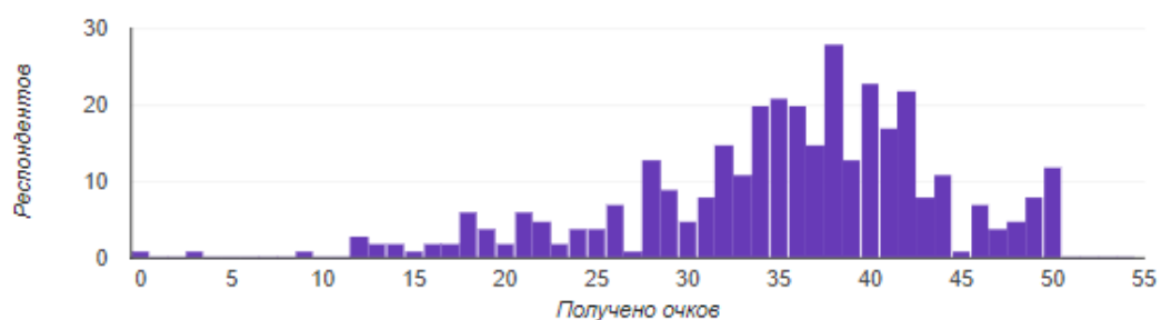
Распределение баллов
