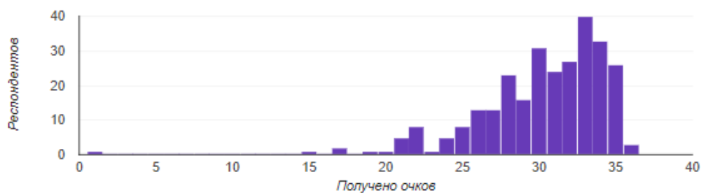
Распределение баллов
