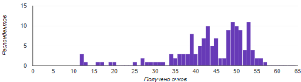
Распределение баллов
