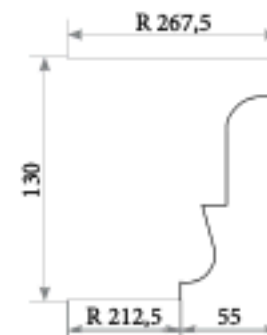
KL 103k 130×535
