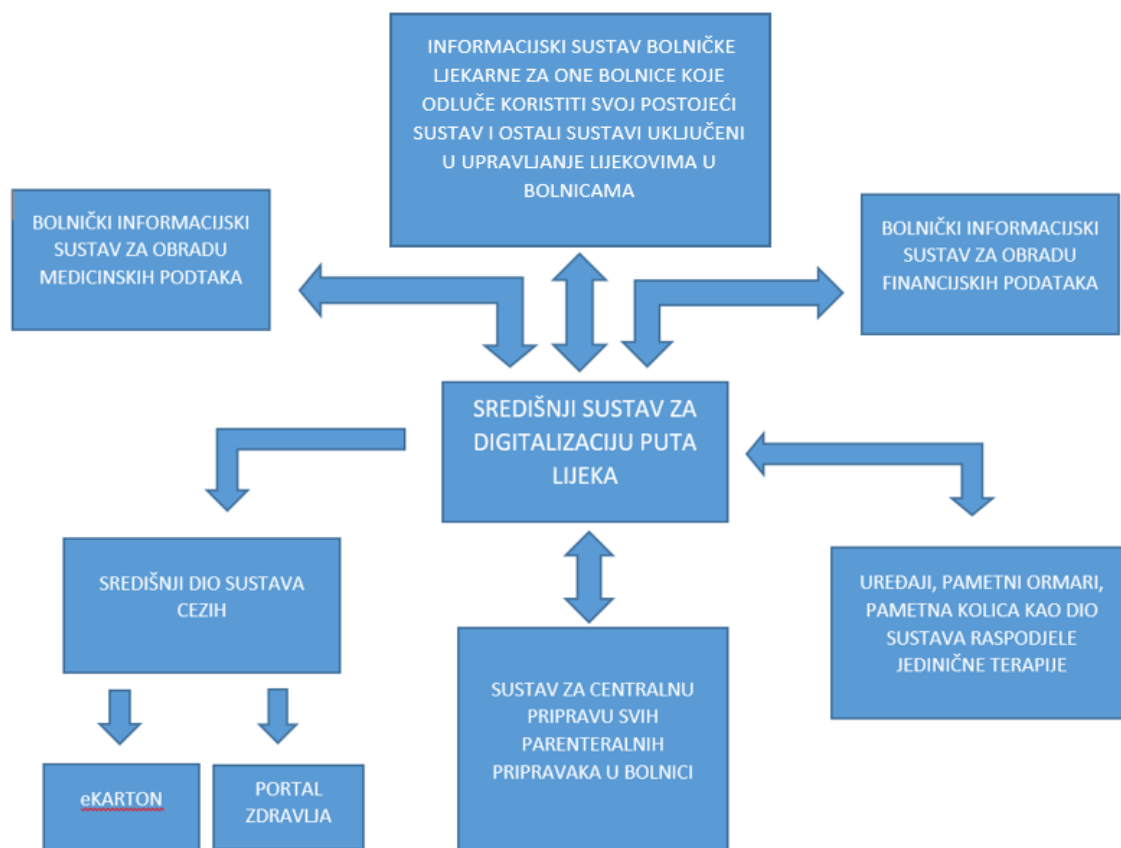
SLIKA 1. Potrebne integracije središnjeg sustava za digitalizaciju puta lijeka s drugim sustavima
