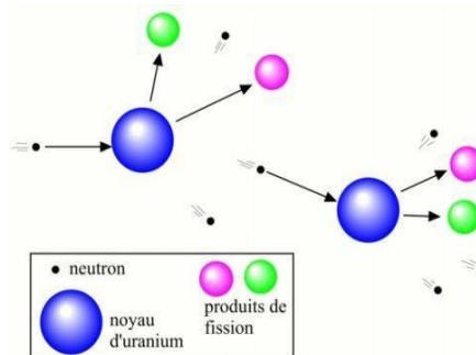
Figure 3 : Réaction en chaîne de fission
