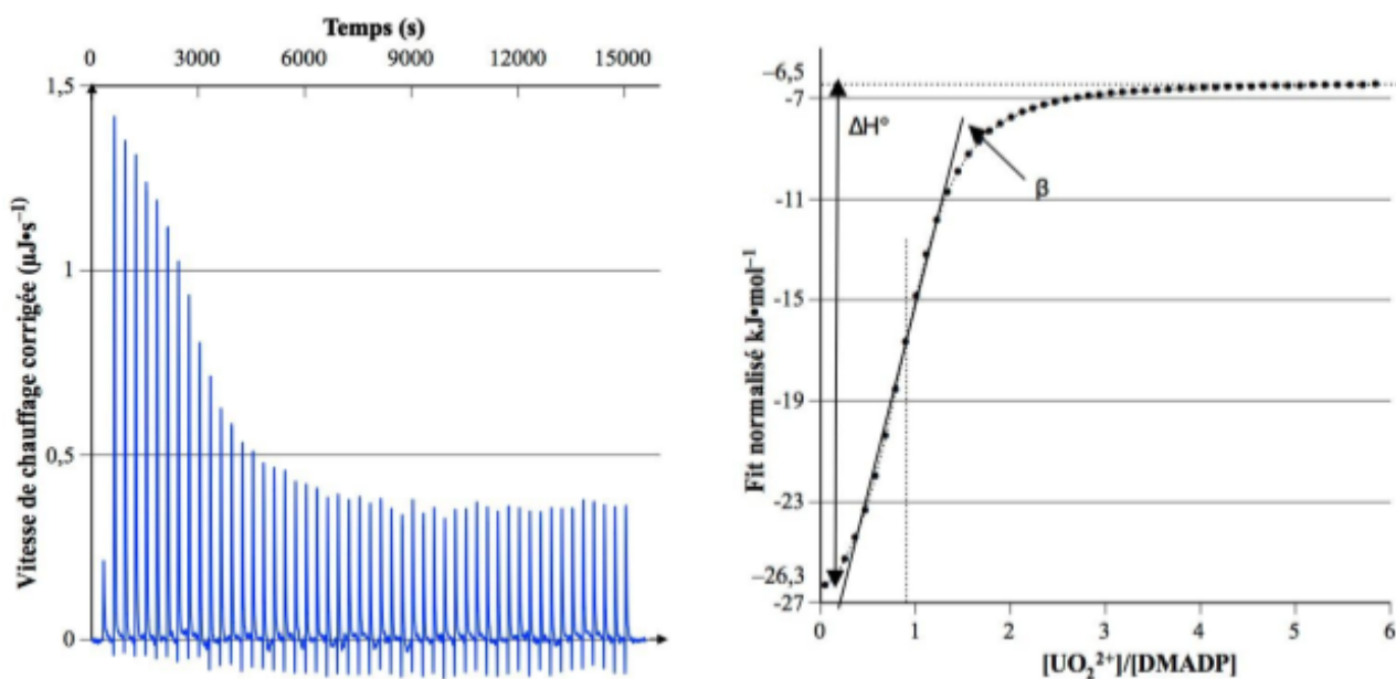
Figure 10 : Thermogramme de l'interaction entre la DAMDP et l'uranyle (à gauche) ; fit de la chaleur dégagée (ou absorbée) en fonction du rapport molaire [\text{cation}]_{\text{total}}/[\text{ligand}]_{\text{total}} (à droite)
