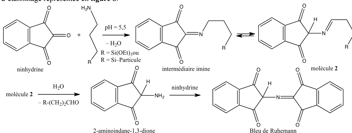
Figure 7 : Réaction de la ninhydrine avec la fonction amine primaire de l'APTES ou avec les fonctions amines présentes sur la surface des nanoparticules une fois qu'elles y ont été fixées
