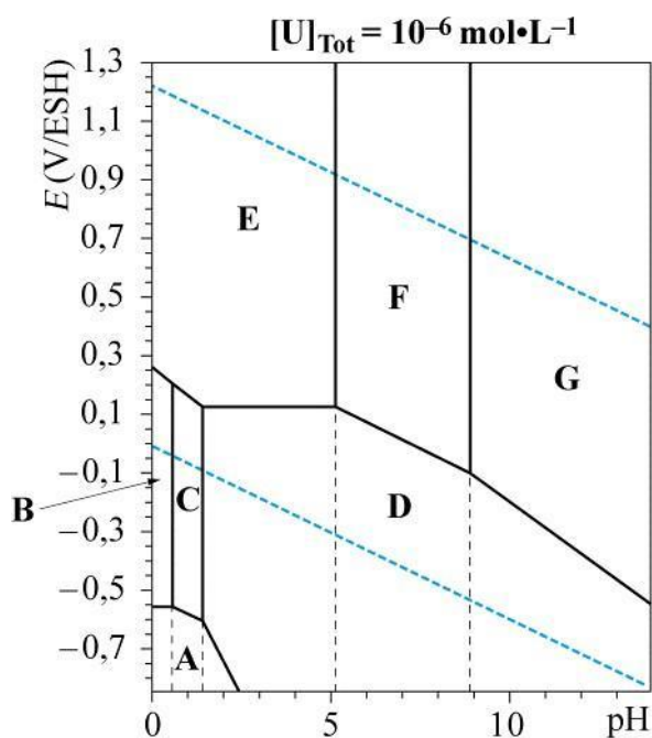
Diagramme potentiel-pH simplifié de l'uranium à 298 K pour une concentration des espèces dissoutes égale à 10^{-6} \text{ mol}\cdot\text{L}^{-1}
