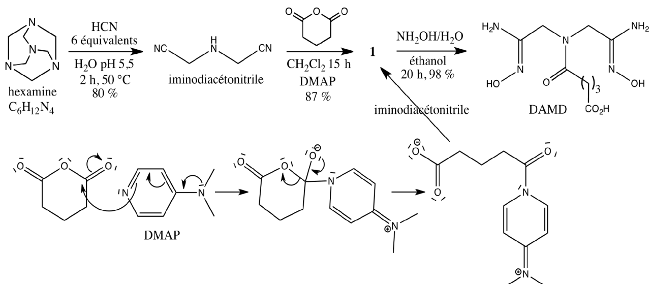
Figure 4 : Synthèse de la DAMD à partir de la molécule d'hexamine et rôle d'activation catalytique de la molécule de DMAP
