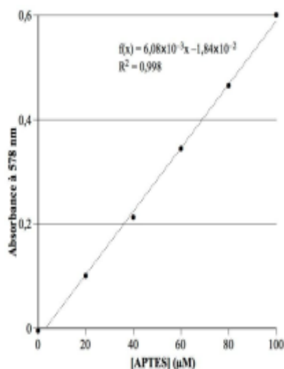
Figure 8 : Courbe d'étalonnage donnant l'absorbance du complexe obtenu à partir d'APTES de concentration connue en μmol.L -1 d'une solution de molécules
