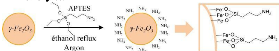
Figure 5 : Traitement de la surface des nanoparticules de maghémite par réaction avec le 3-aminopropyltriéthoxysilane
