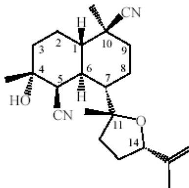
Kalihinol C
