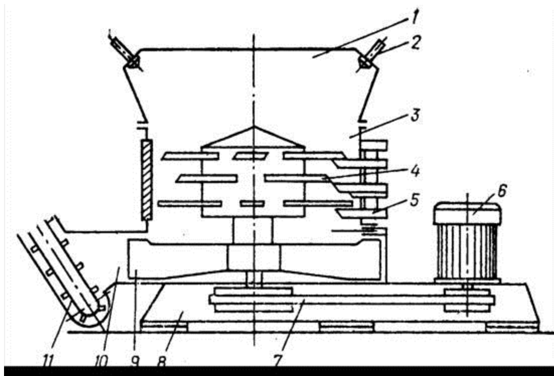
Рис. 3. Конструктивна схема подрібнювача-змішувача кормів ИСК-3А:
