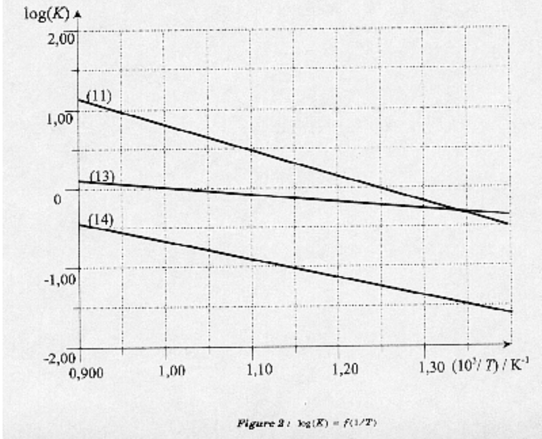
Fig. 2. \log K(T) = f(\frac{1}{T}) ). Cette figure est à rendre avec la copie.
