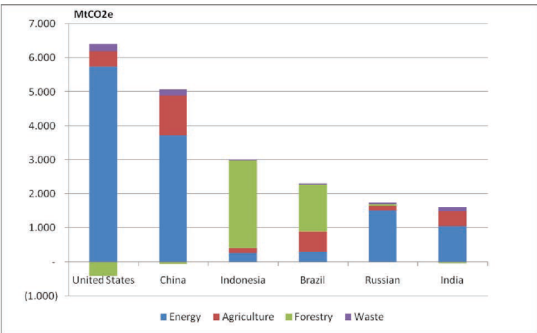
Gambar 1 Emisi Gas Rumah Kaca di Beberapa Negara
