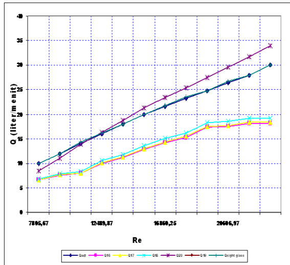
Gambar 10. Grafik perbandingan Q_{\text{aktual}} dengan Q_{\text{teoritis}} dan Q_{\text{sightglass}} pada beberapa posisi pengukuran \Delta P orifis rasio diameter 0.7 dan tebal 10 mm
