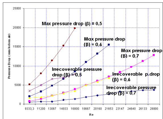
Gambar 13. Grafik maximum pressure drop dan irrecoverable pressure drop orifice flow meter dengan tebal orifice plate 10 mm
