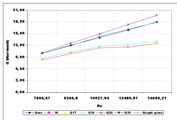
Gambar 12. Grafik perbandingan Q_{\text{aktual}} dengan Q_{\text{teoritis}} dan Q_{\text{sightglass}} pada beberapa posisi pengukuran \Delta P orifis rasio diameter 0.5 dan tebal 10 mm
