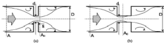
Gambar 1. Profil aliran melewati plat orifice tipis dan tebal
