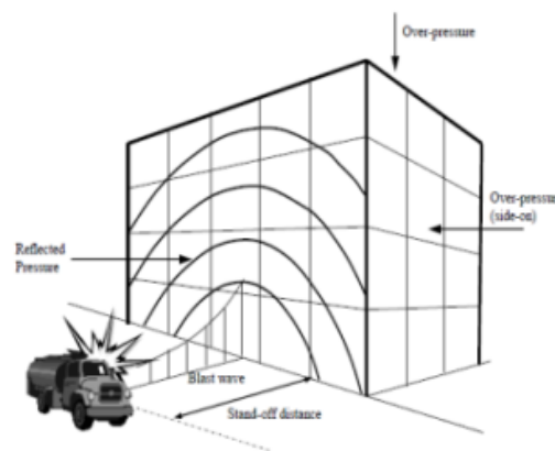
Gambar 1. Simulasi Ledakan Kendaraan
