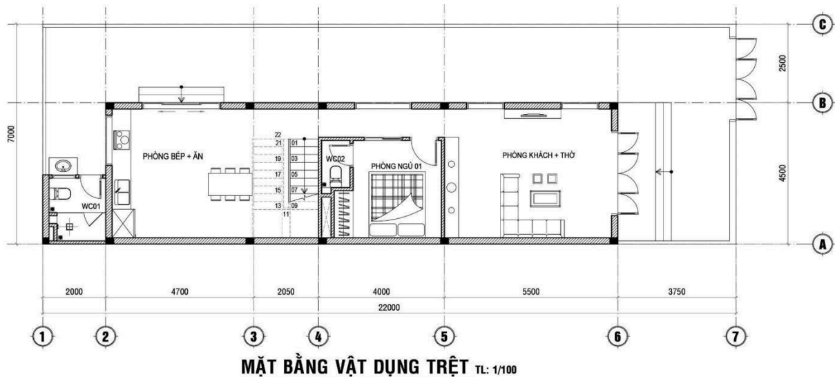
Bản vẽ thiết kế tầng trệt của nhà anh Dũng (mb1)
