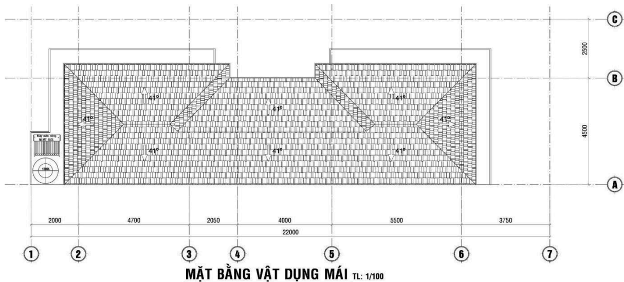
Bản vẽ thiết kế mái của nhà anh Dũng (mb3)
