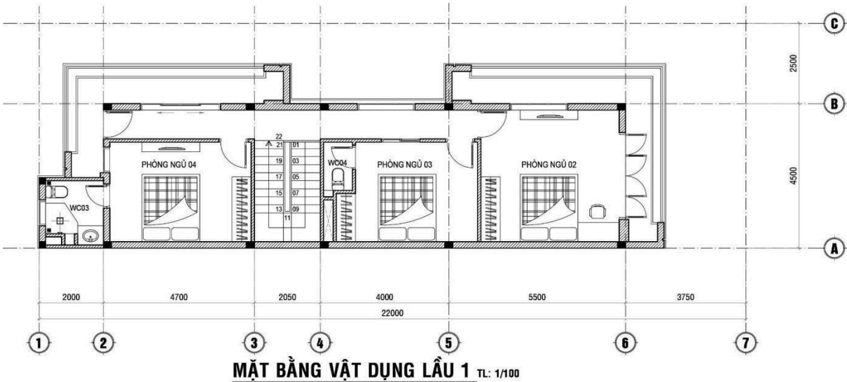
Bản vẽ thiết kế lầu 1 của nhà anh Dũng (mb2)
