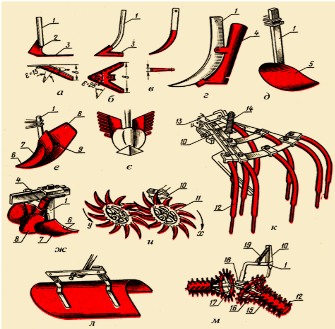
Рис. 1.5.9. Робочі органи культиваторів:
