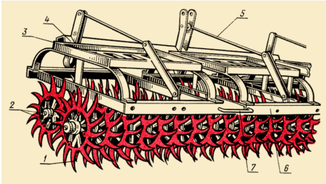
Рис. 2. Ротаційна мотика МНВ-2,8
