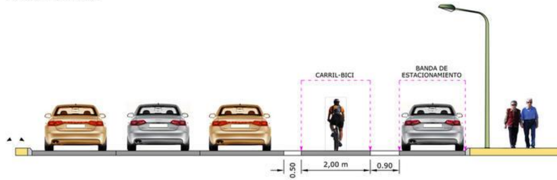
Sección A (Carril-Bici)
