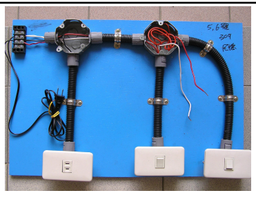
室內配線基礎配電盤
