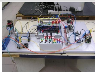
基礎氣壓控制實習盤
