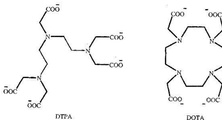
Figure 1 : Structure des ligands DTPA et DOTA.
