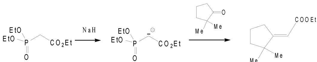
Figure 1 : exemple de réaction de Horner-Wadsworth-Emmons.
