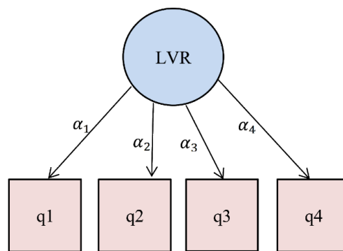
Gambar 1. Jalur SEM-PLS
