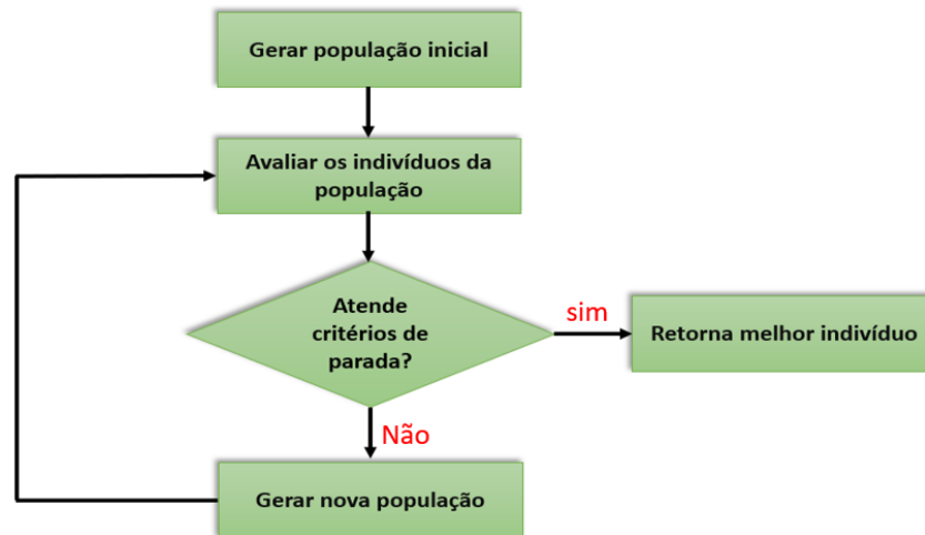
Figura 3.1- Fluxograma PG básico
