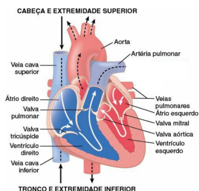
Figura 2.1- Estrutura simplificada do coração
