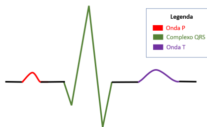
Figura 1.1- Representação das ondas do sinal de ECG
