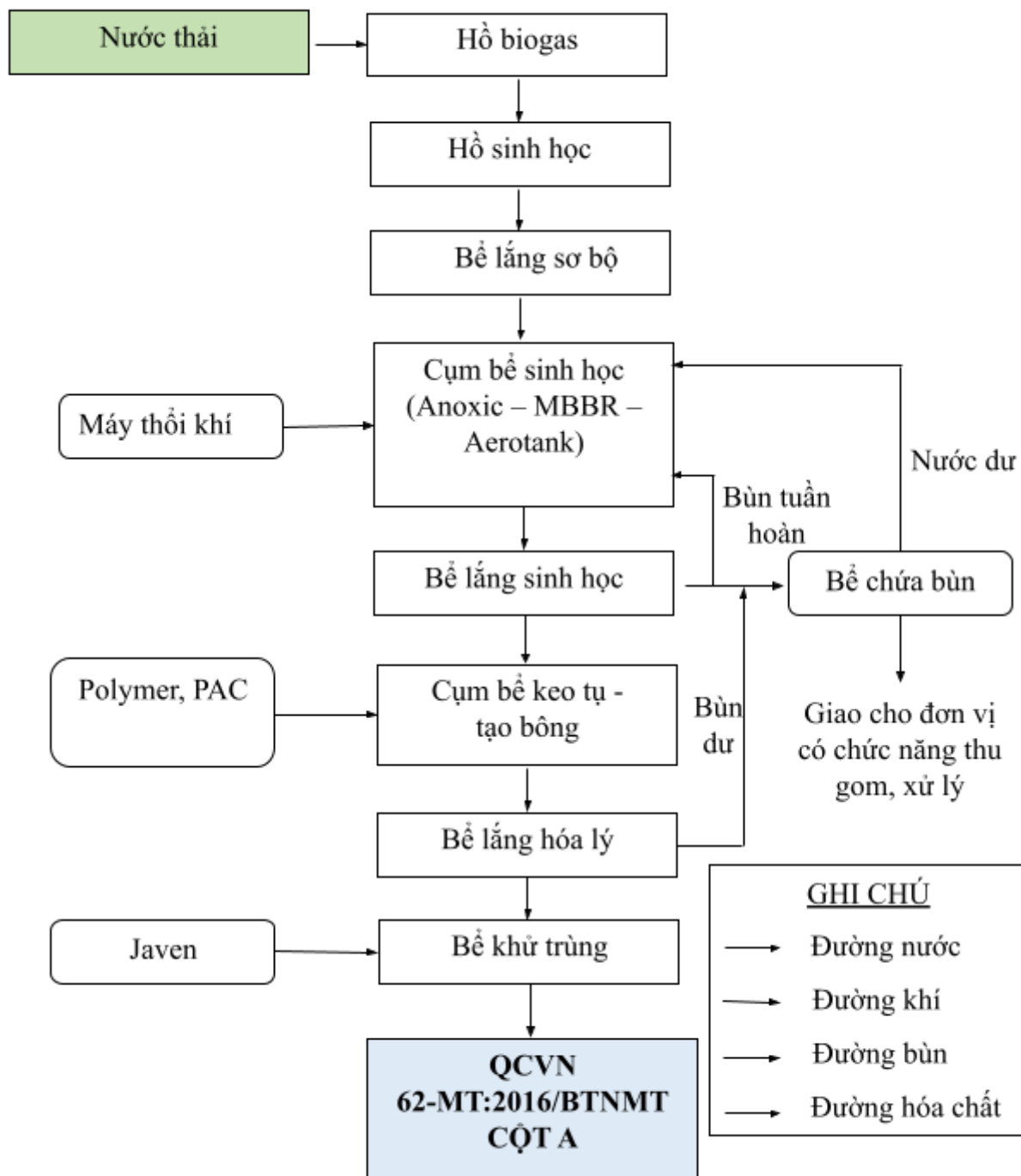
Sơ đồ quy trình HTXLNT, công suất 200 m 3 /ngày.đêm của Trại Đỗ Minh Tuấn
