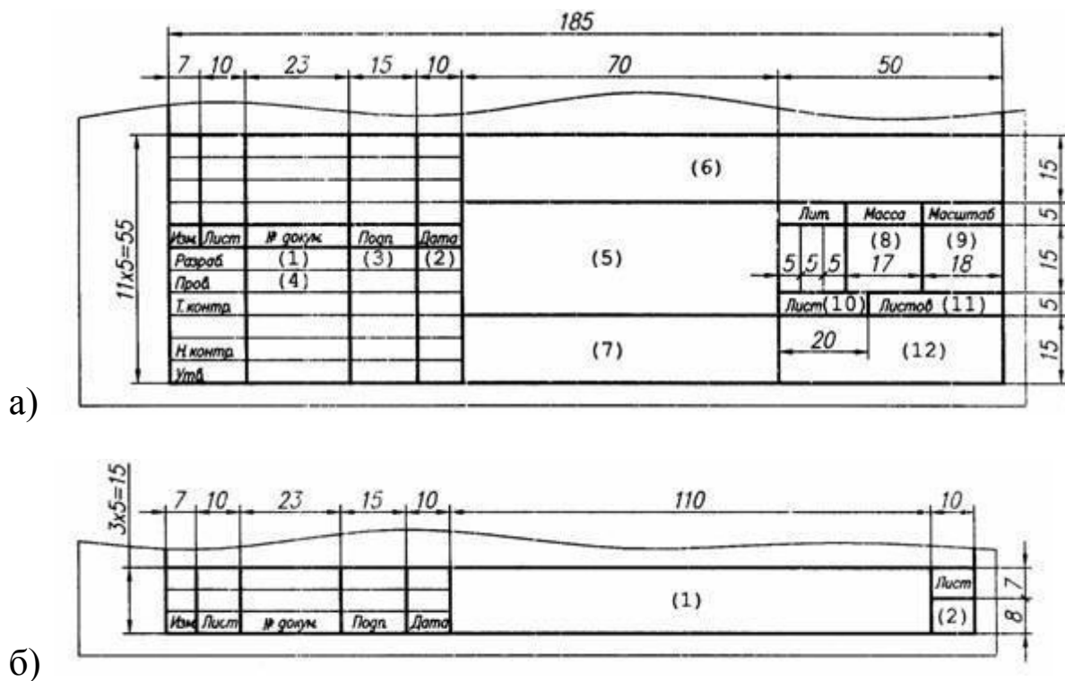
Рис. 2. Основний напис креслення: а — форма 1; б — форма 2а
