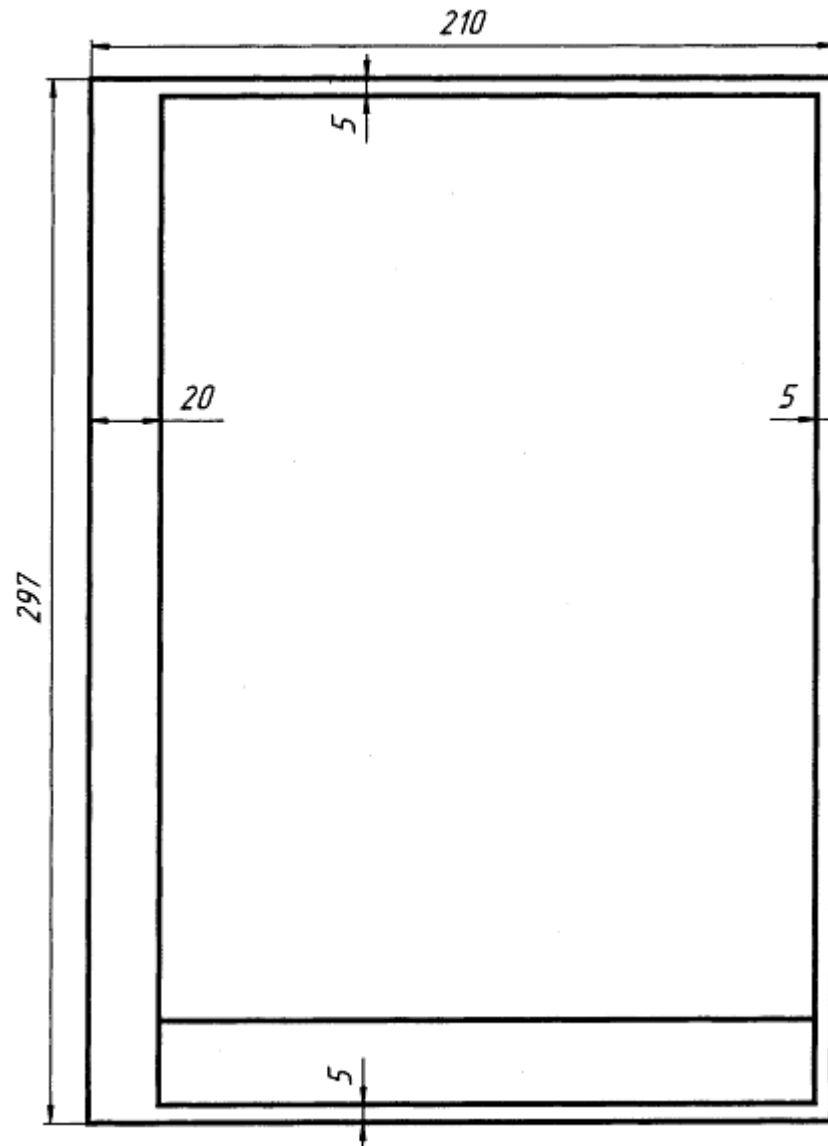
Рис. 1. Оформлення аркуша креслення формату А4
