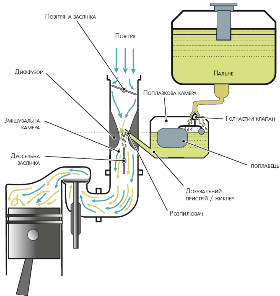
Малюнок 4.47б Найпростіший карбюратор.
