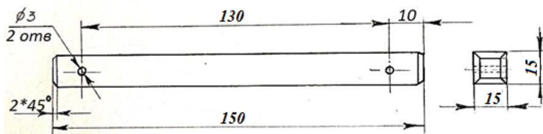
Деталь 2( 16 шт.)
