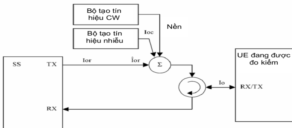
Hình C.5 - Sơ đồ đo kiểm RX với cả nhiễu và CW bổ sung
