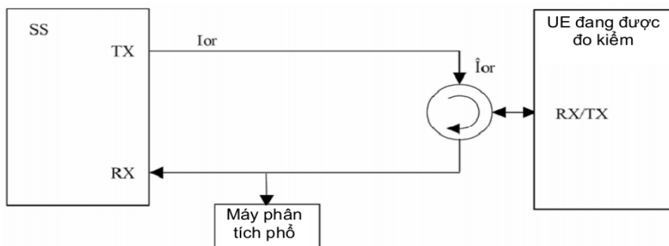
Hình C.6 - Sơ đồ đo kiểm phát xạ giả
