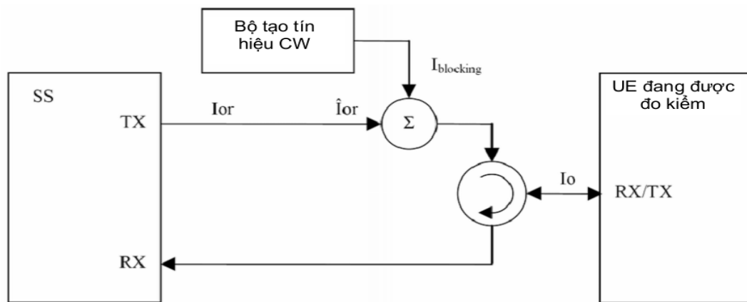
Hình C.4 - Sơ đồ đo kiểm RX với CW bổ sung
