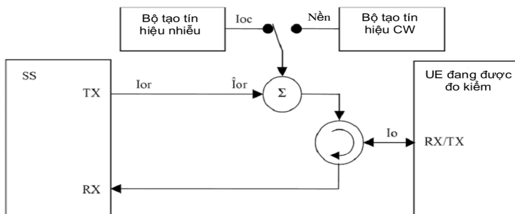
Hình C.3 - Sơ đồ đo kiểm RX với nhiễu hoặc CW bổ sung
