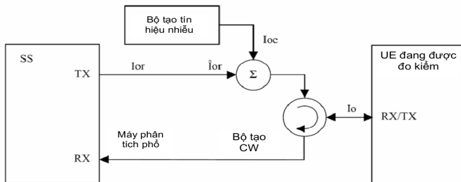
Hình C.2 - Sơ đồ đo kiểm RX với nhiễu
