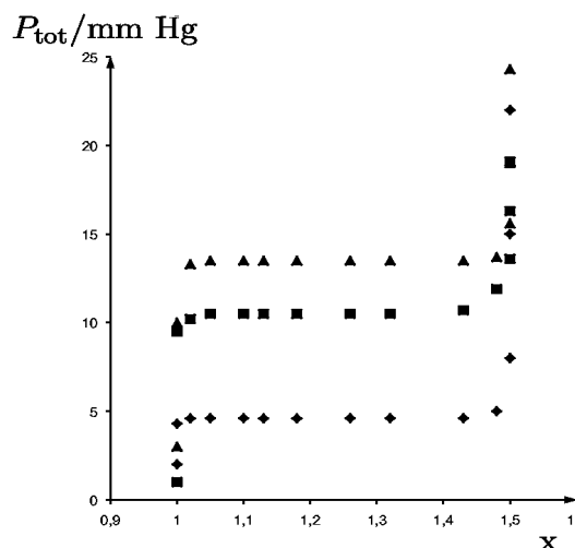
Figure 5. Courbe isotherme représentant la variation de la pression p_\text{tot} en fonction du paramètre de composition x représentant le rapport m_\text{S}/m_\text{D} . ♦ : expérience réalisée à 9, 7°C. ■ : expérience réalisée à 21, 6°C. ▲ : expérience réalisée à 25, 4°C.
