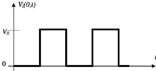
Figure 3 : Onde incidente
