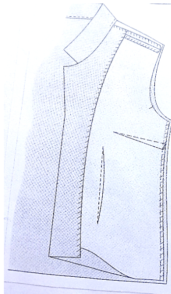
Montáž bočných švov
