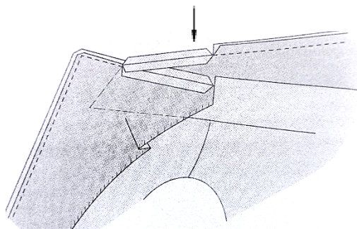
Rozžehlené švy všítia goliera
