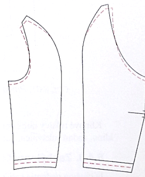
Obr. Oprava strihu klinových rukávnic
