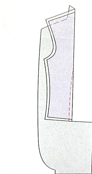
Odšitie predného priestrihového odševku
