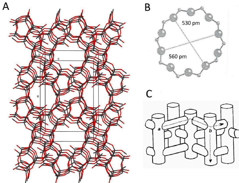
Figure 4 : (A) Structure de la zéolithe ZSM-5 (type MFI) ; les cations ne figurent pas sur la figure pour mieux montrer la porosité. (B) Détail des fenêtres des pores, d'après l'"Atlas of Zeolite Framework Types". (C) Système de canaux de la zéolithe ZSM-5 : un sinusoïdal (a) et l'autre droit (b).
