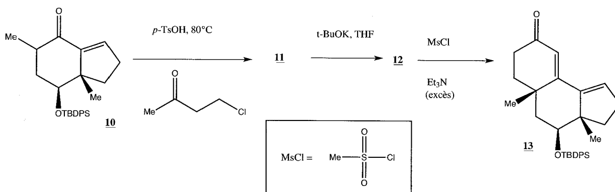
Figure 15 : Synthèse de 13 à partir de 10 .
