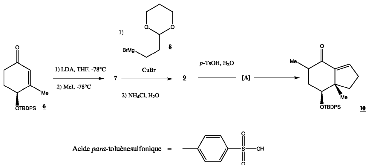
Figure 13 : Synthèse de 10 à partir de 6 .
