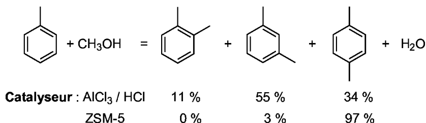
Figure 7 : Méthylation du toluène.
