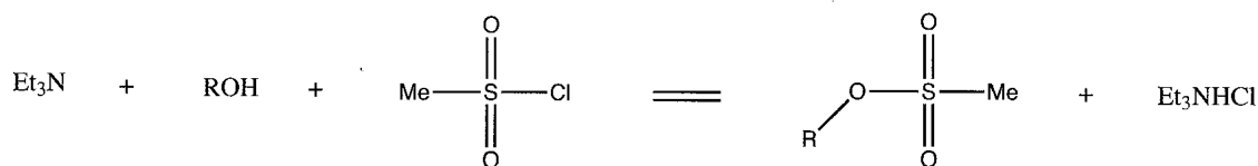
Figure 16 : Action du chlorure de méthanesulfonyle sur un alcool en présence de triéthylamine.
