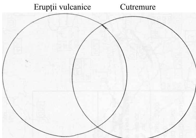
Diagrama Venn
