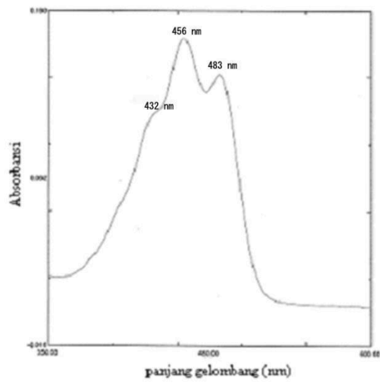
Gambar 1. Spektrum UV senyawa hasil isolasi dalam n-heksan
