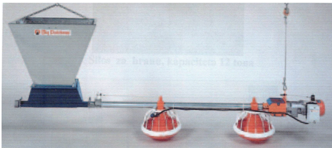
Аутоматски систем храњења и појења
