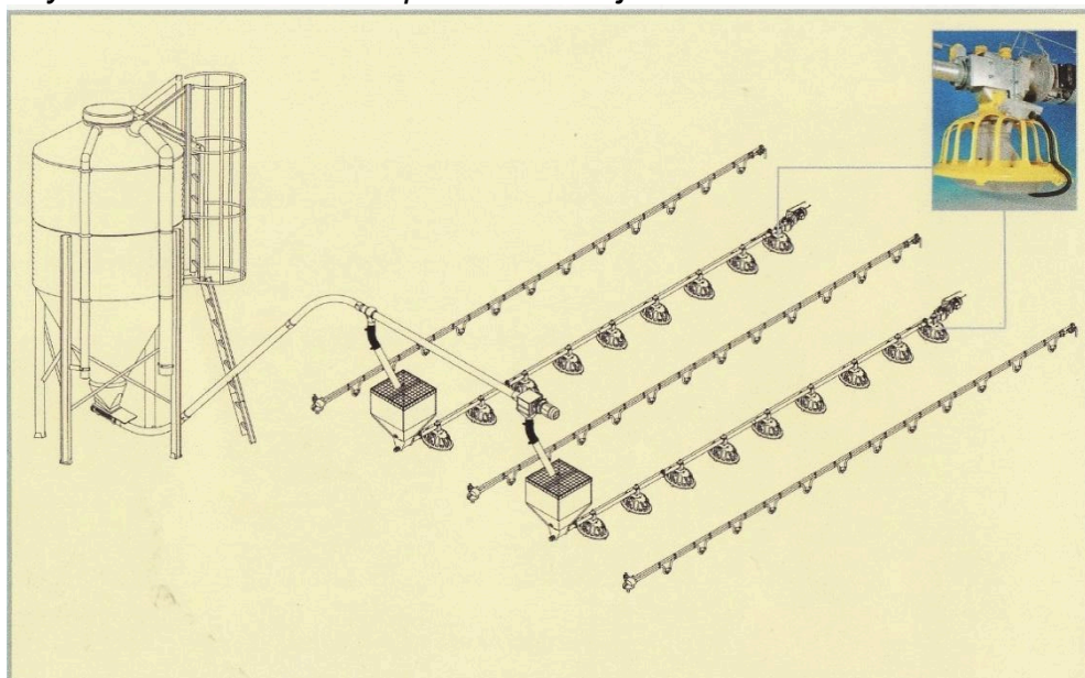
Аутоматски систем храњења и појења
