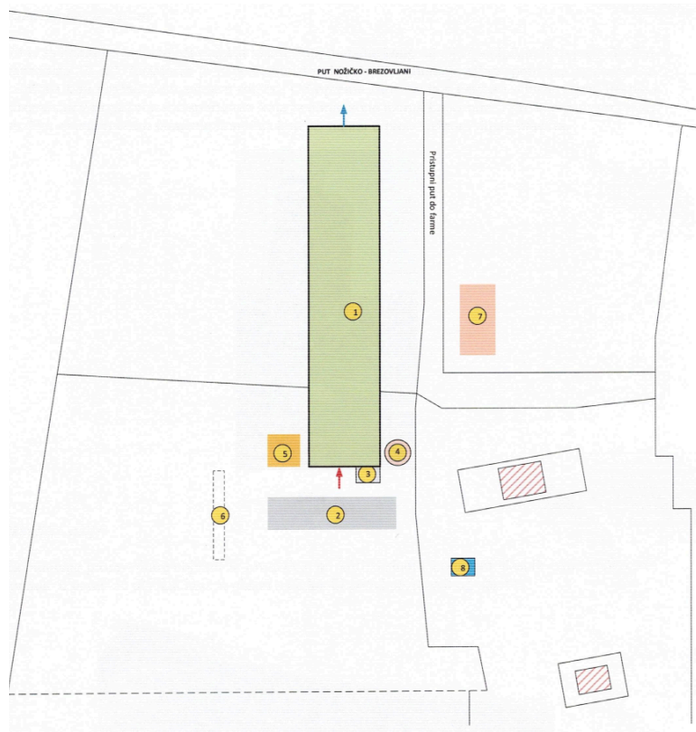
Основа објекта за тов бројлера
