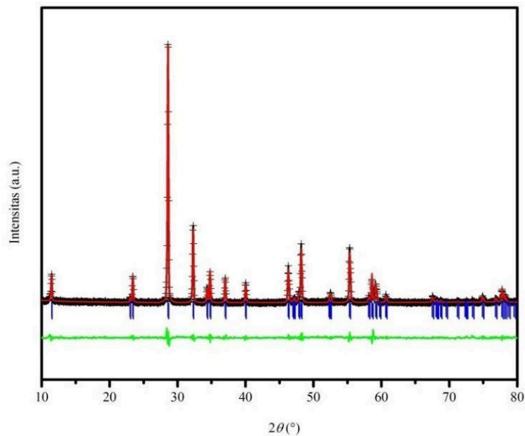
Gambar 4 Plot hasil refinement pola difraksi sinar-X serbuk oksida \text{Bi}_2\text{Zn}_{0,1}\text{V}_{0,9}\text{O}_{5,35} setelah dibakar pada suhu 600 °C selama 24 jam. Tanda + yang berwarna hitam merupakan data pengamatan hasil difraksi sinar-X, garis merah adalah hasil kalkulasi, garis vertikal warna biru adalah posisi Bragg yang diharapkan, garis hijau adalah perbedaan antara hasil kalkulasi dan data pengamatan difraksi sinar-X (perbedaan antara tanda + berwarna hitam dan garis merah).
