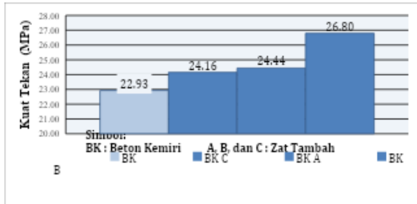
Gambar 1. Hasil Pengujian Kuat Tekan Beton Variasi
