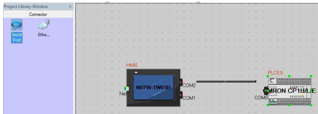
Hình 2.6. Tạo liên kết giữa PLC và HMI qua cổng truyền thông RS485.
