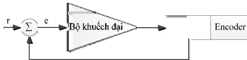
Hình 2.17. Điều khiển động cơ servo chế độ mạch vòng kín.
