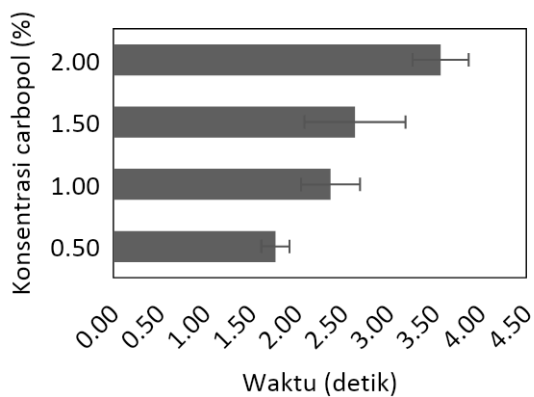
Gambar 1. Hasil uji daya lekat gel serbuk lidah buaya ( Aloe vera L. ) berbasis carbopol 934
