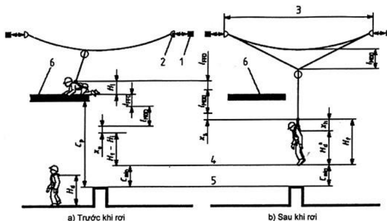
Hình 1 - Các bộ phận của dây cứu sinh ngang
