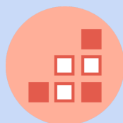
Periodic Table
