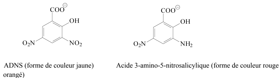
Figure 6. Formules de l'ADNS et de l'acide 3-amino-5-nitrosalicylique
