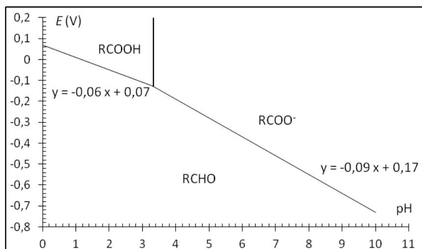
Figure 3. Diagramme potentiel-pH simplifié du glucose (noté RCHO).
