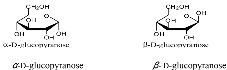
Figure 5. Formule des formes cycliques du glucose
