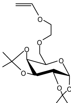
Figure 11. Formule du monomère 1,2:3,4-di- O -isopropylidene-6- O -(2-vinyloxyethyl)- \alpha -D-galactopyranose (noté GVE)
