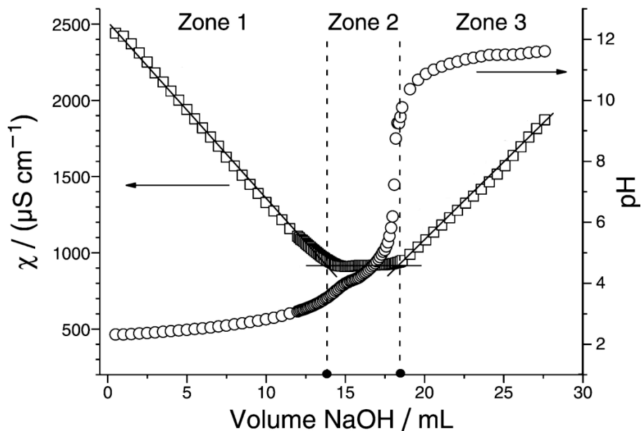
Figure 8. Courbes de titrage de l'homogalacturonane réalisé par pH-métrie (●) et conductimétrie (□). On précise que la zone 2 correspond à 14,0 \text{ mL} < V_{\text{NaOH}} < 17,9 \text{ mL}
