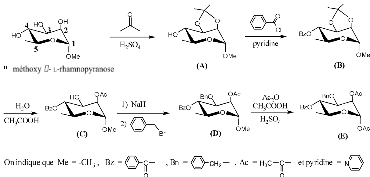
Figure 9. Schéma de synthèse d'un dérivé du méthoxy \alpha -L-rhamnopyranose.
