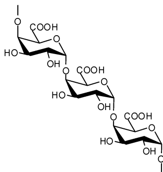
Figure 7. Formule du fragment homogalacturonane d'une pectine
