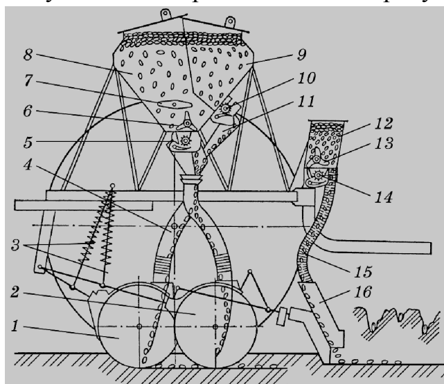
Рис. 2.7. Функціональна схема зернотукотрав'яної сівалки СЗТ-3,6А: 1 і 2 — дискові сошники; 3 — штанги з пружинами; 4 і 15 — насіннепроводи; 5 і 14 — насінневисівні апарати; 6 і 13 — нагнітачі; 7 — ворушилка; 8 і 9 — відділення ящика зернотрав'яне і для добрив; 10 — туковисівний апарат; 11 — лотік; 12 — ящик для насіння трав; 16 — кілеподібний сошник
