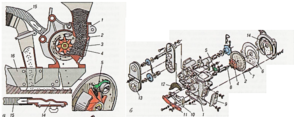
Рис. 4.9. Дисківий пневматичний висівний апарат сівалки СУПН-8А:
