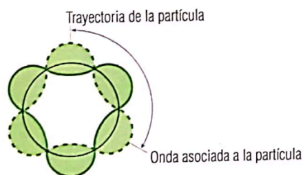
Relación entre una partícula en movimiento y su onda asociada.
