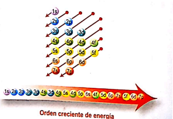
Regla de las diagonales.
