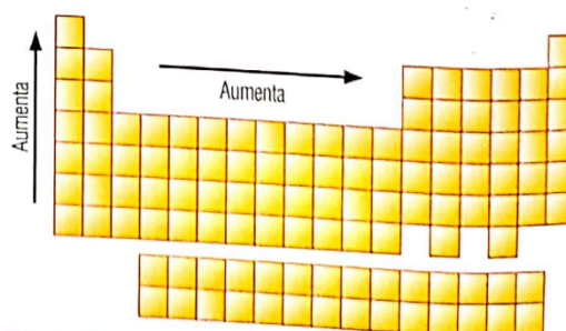
Variación de la energía de ionización en la tabla periódica.
