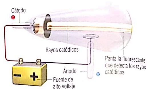
Esquema de un tubo de rayos catódicos similar al construido por Thomson.
