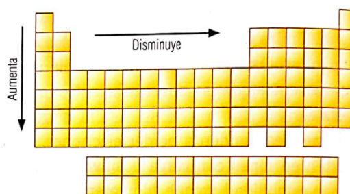
Variación del radio atómico en la tabla periódica.
