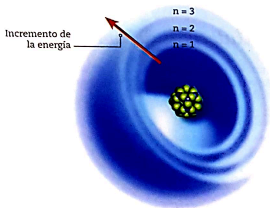
Modelo atómico actual: se advierten zonas u orbitales donde es posible encontrar a los electrones.
