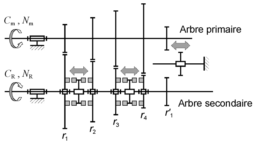
Figure 10 : Schéma d'une boîte de vitesses
