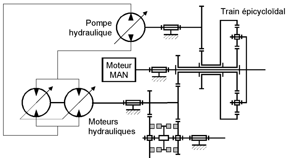
Figure 14 : Schéma cinématique de la transmission Fendt
