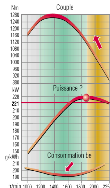
Figure 4 : Courbes caractéristiques
