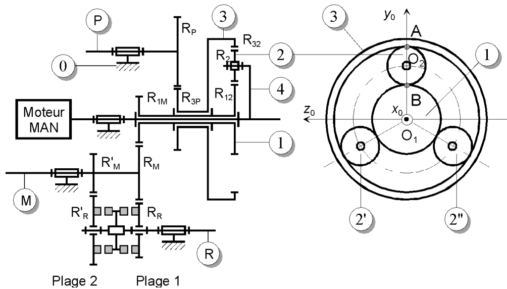
Figure 15 : Partie mécanique de la transmission Vario
