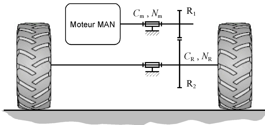
Figure 9 : Réducteur à un étage
