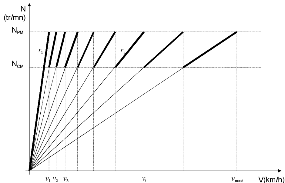
Figure 12 : Evolution de N en fonction de V suivant le rapport r_i de transmission
