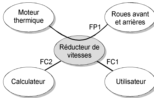
Figure 5 : Diagramme partiel des interacteurs d'un réducteur de vitesses
