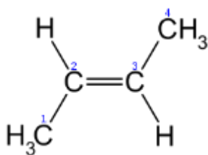
транс-2-бутен
