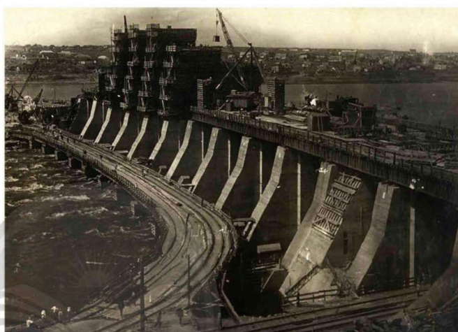
1.8 Nhà máy thủy điện Đni-ép (Dnepr) được xây dựng năm 1927 Đây là đập thủy điện lớn nhất châu Âu đương thời và được ca ngợi là một trong những thành tựu lớn nhất của chương trình công nghiệp hoá Liên Xô.
