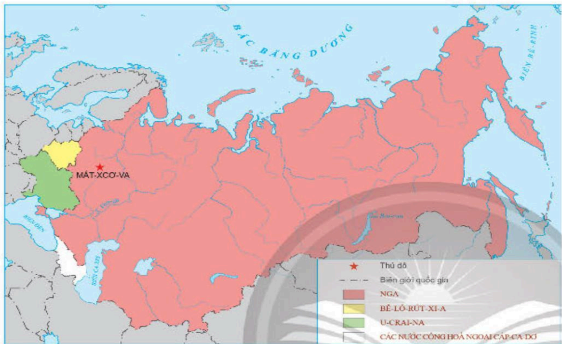
1.3 Lược đồ Liên Xô năm 1922
