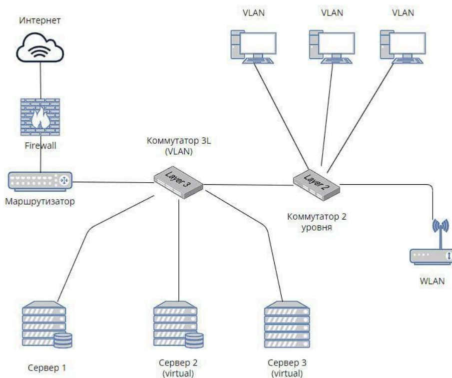
Рис.1. Схема сети
